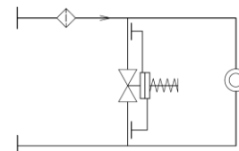
Установка регулятора на перепадке
