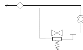
Установка регулятора на обратном трубопроводе
