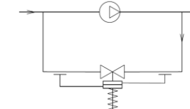
Установка регулятора на байпасе насоса
